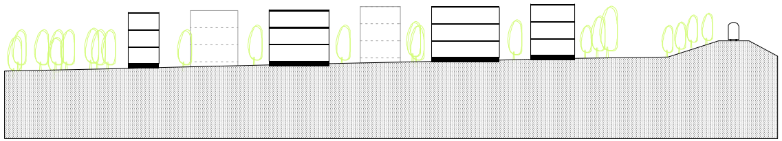
snede A_A
